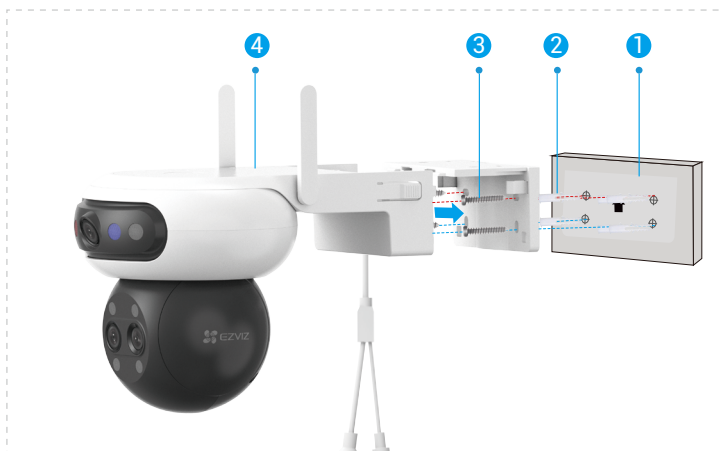
Rys. 2 Montaż ścienny
